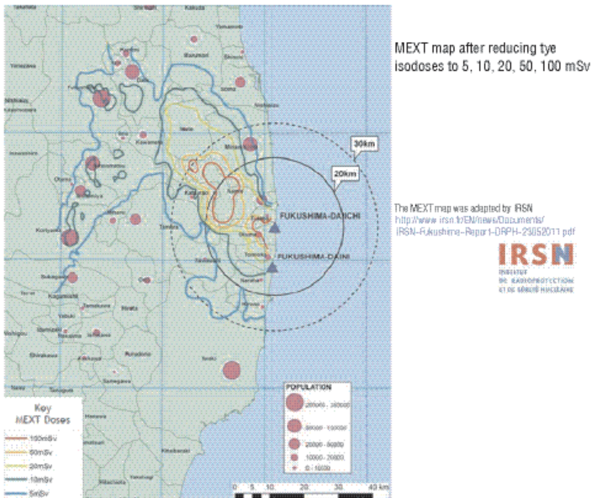
Рис. 6. Оценка годовых доз внешнего облучения, по данным MEXT.
